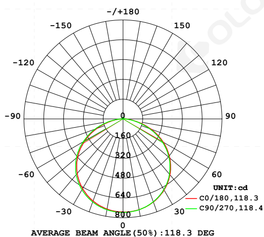
配光曲线图
